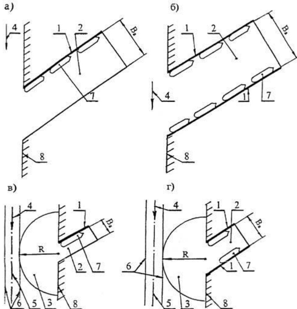
Рисунок 4.4.2 - Схема акваторий причалов и водных подходов к ним при расположении причалов в русле реки
