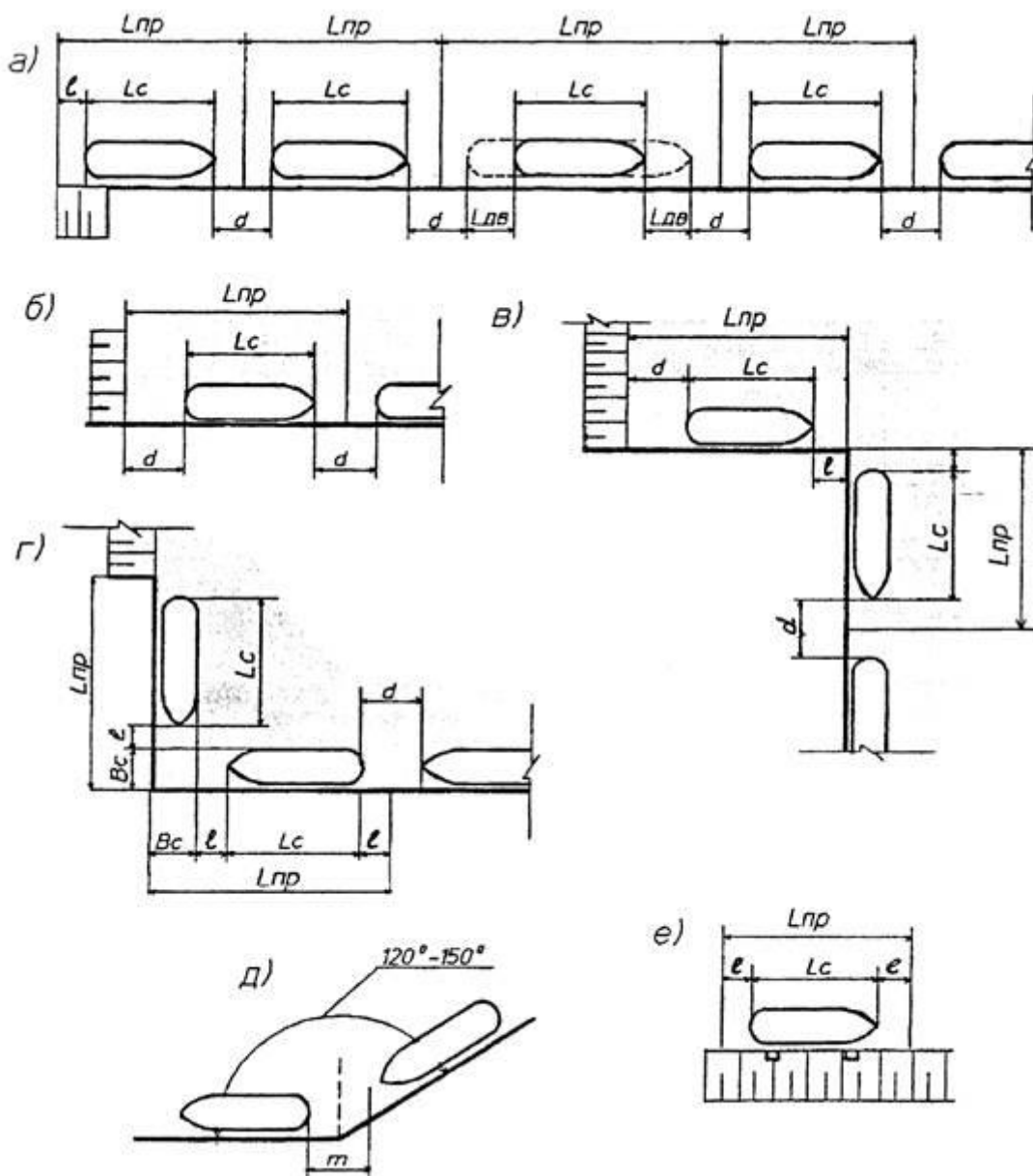
Рисунок 4.5.1 - Схемы размещения судов у причала
