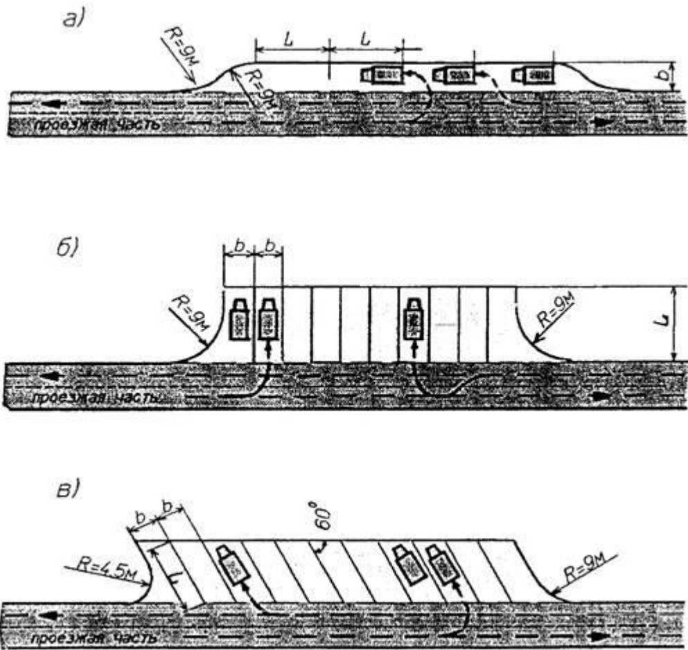
Рисунок 4.4.1 - Схемы площадок для стоянки грузовых автомобилей
