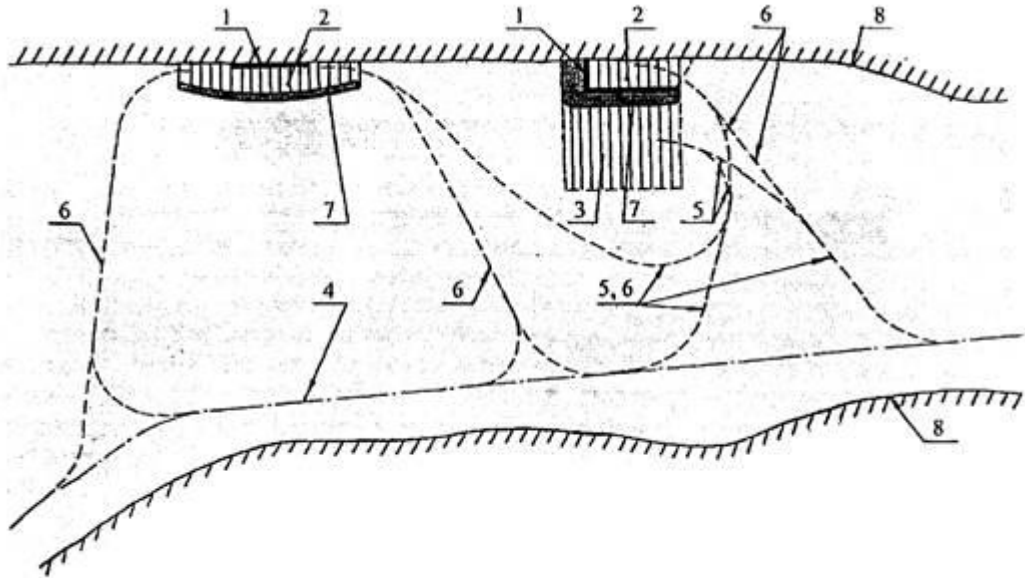
Рисунок 1 - Схема расположения порта на реке
